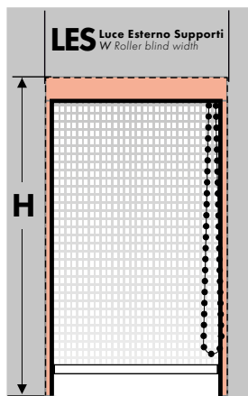
STANDARD DA INTERNO CATENELLA A DESTRA Chain on the right side
