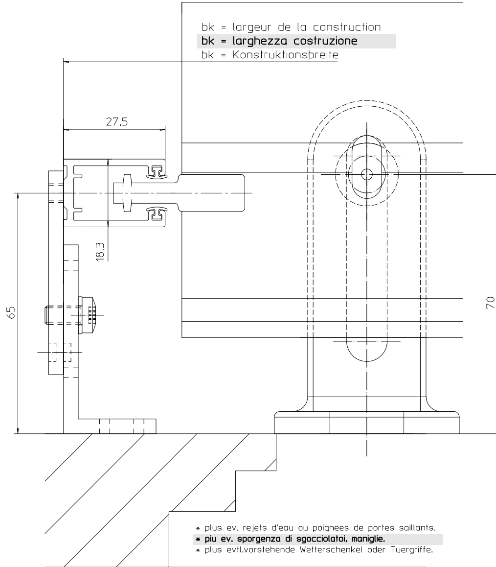
coulisse avec support guida con supporto Fuehrung mit Halter
