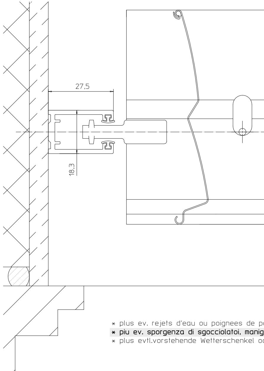
coulisse sur crepi guida su intonaco Fuehrung auf Putz
