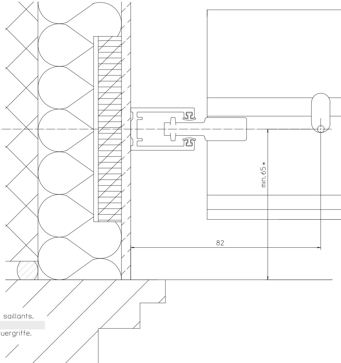
coulisse sur isolation avec vis normales pour chevilles guida su isolamento con viti normali Fuehrung auf Isolation mit Normalschrauben
