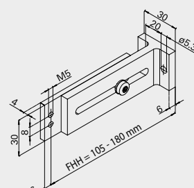
Squadretta per guide tipo 4
