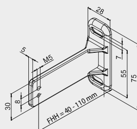
Squadretta per guide in ghisa tipo 2
