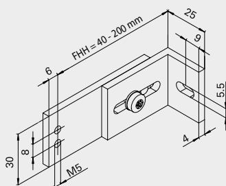
Squadretta per guide FEH tipo 3
